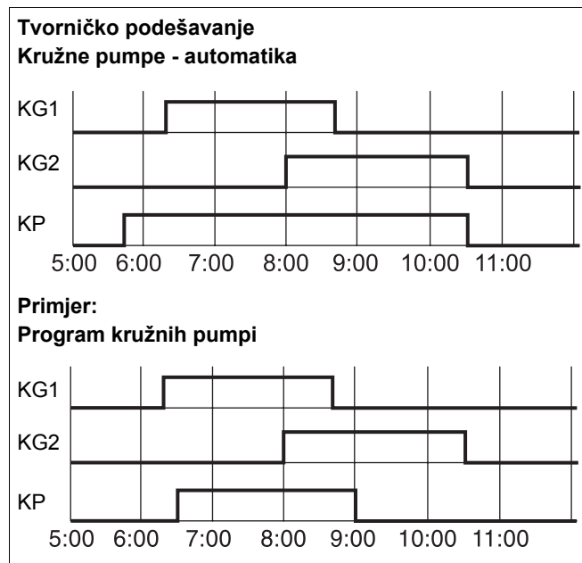
Sl. 11 Unošenje novog programa kružnih pumpi
