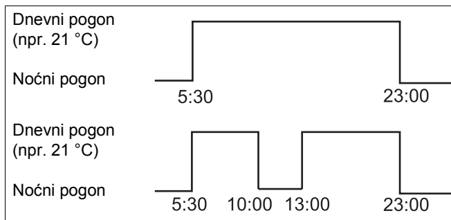
Sl. 7 Zadavanje uklopnih točki
