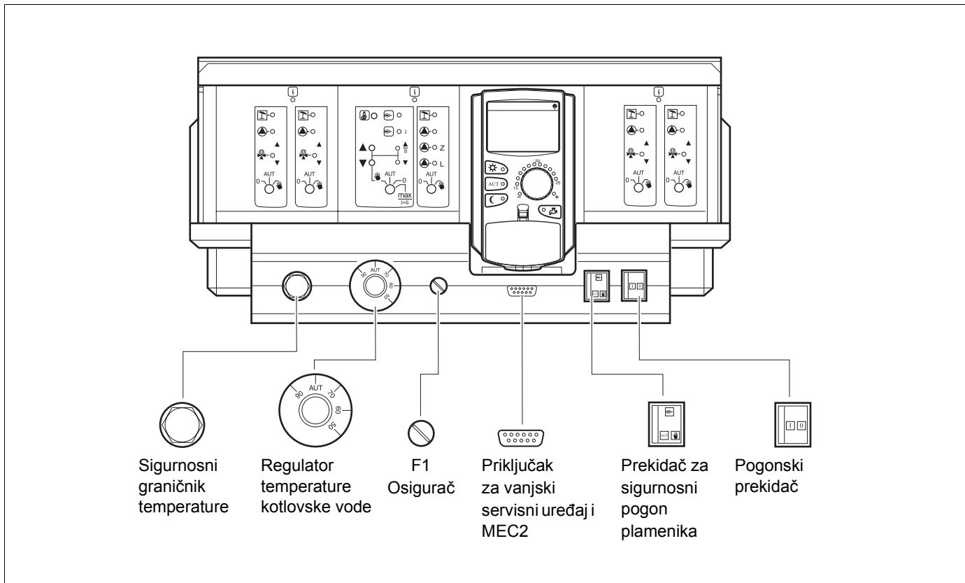
Sl. 1 Poslužni elementi
