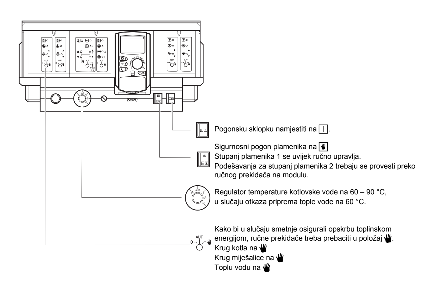
Sl. 13 Pogon grijanja preko ručnog prekidača
