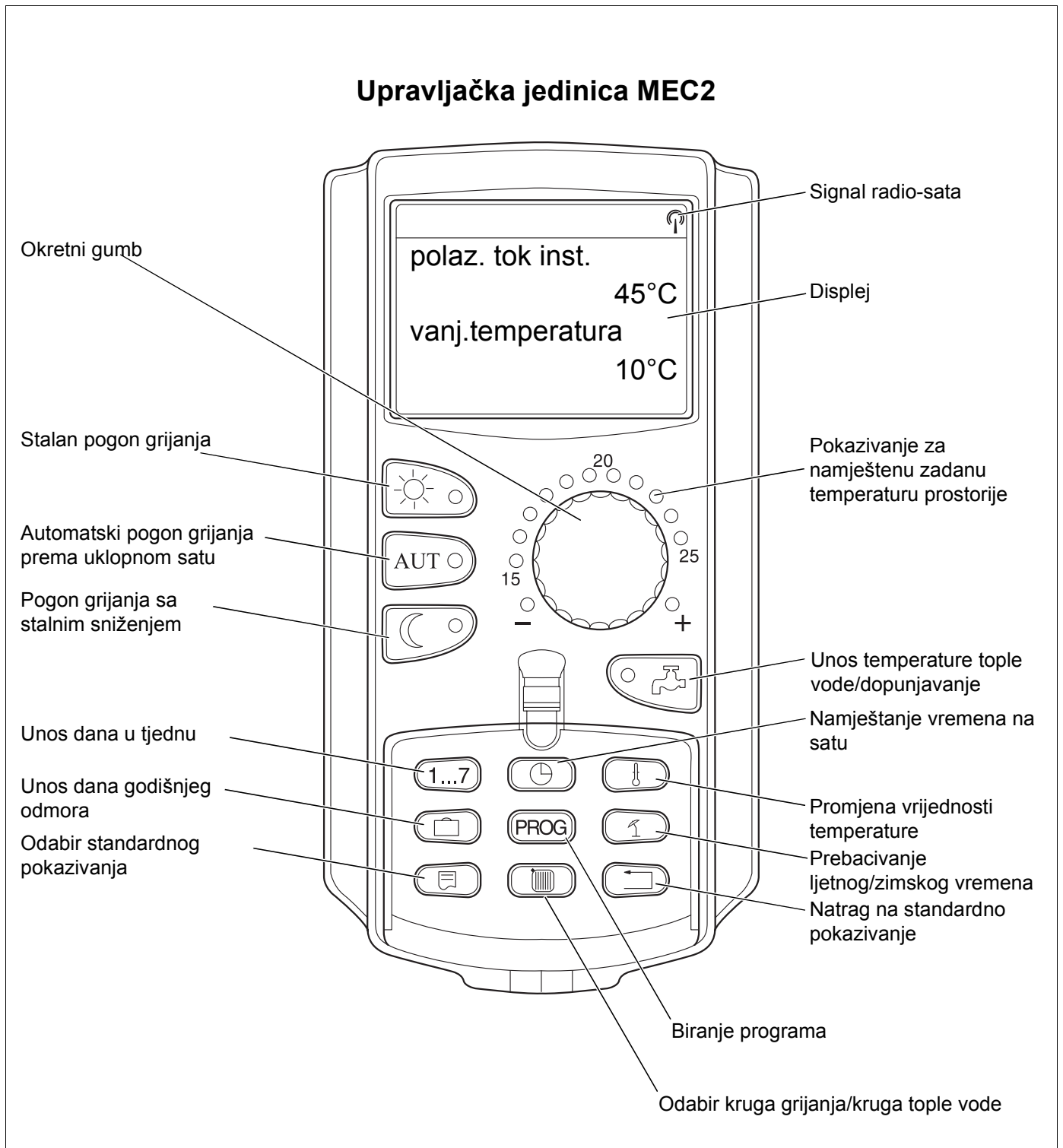
Sl. 5 Upravljačka jedinica MEC2
