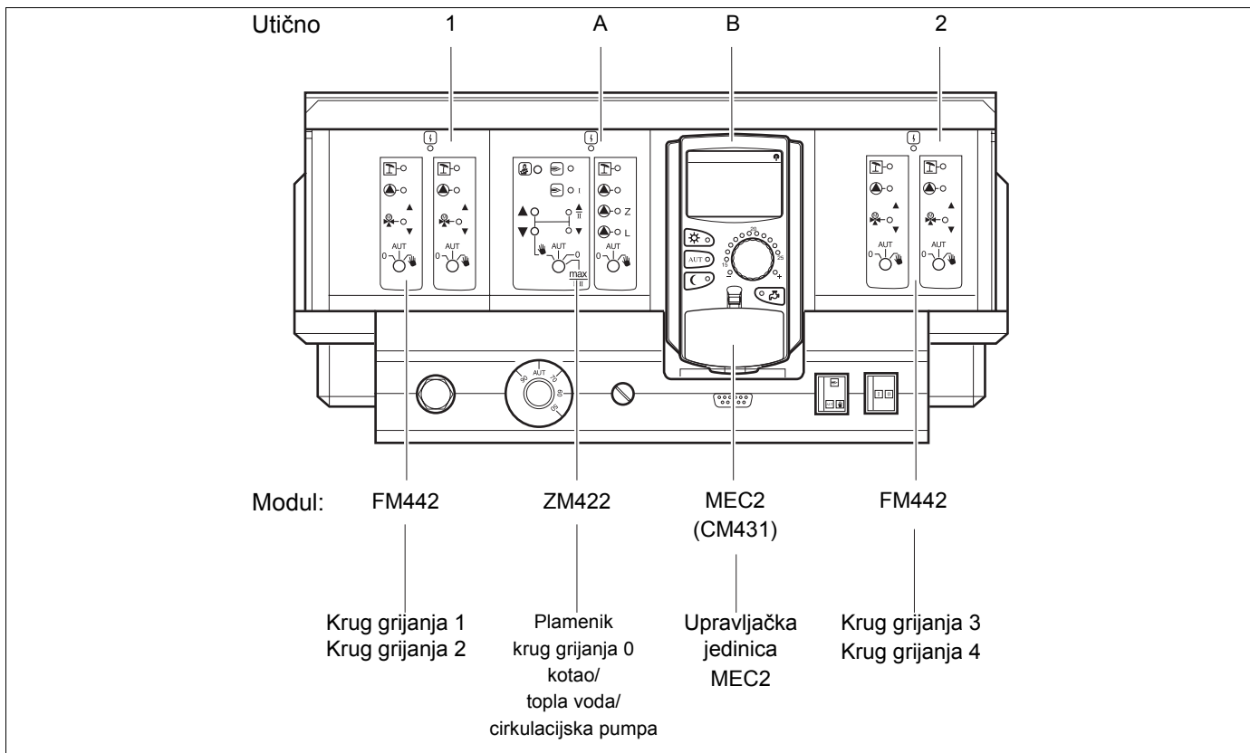
Sl. 2 Opremljenost modula
