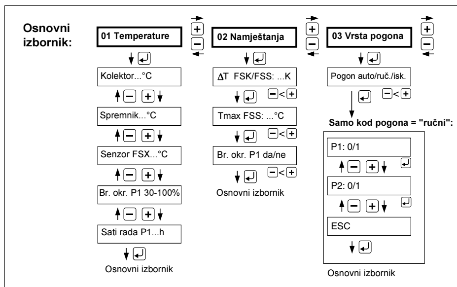
Sl. 4 Vođenje kroz izbornik regulacijskog uređaja
